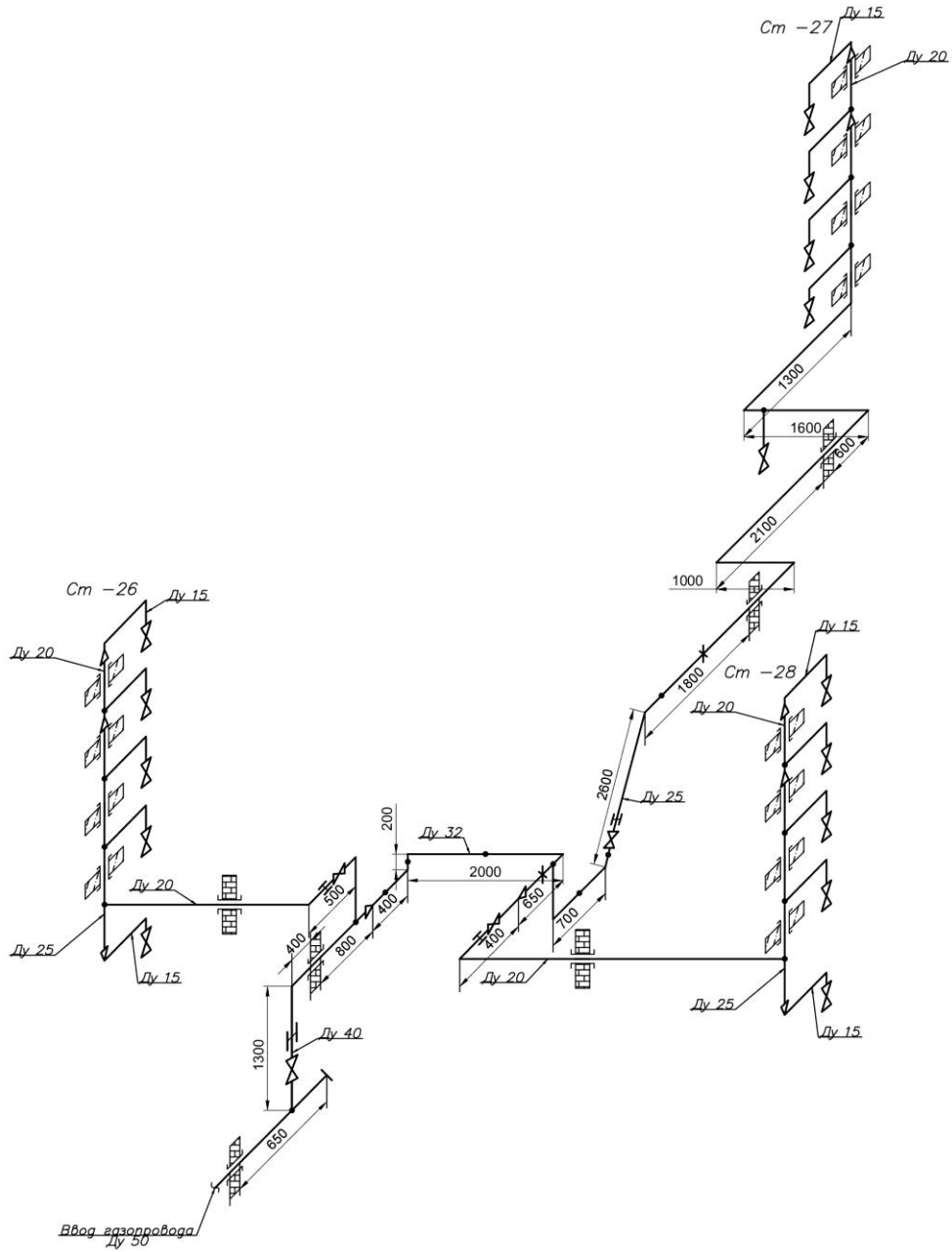
АксонOMETрическая схема внутридомового газового оборудования по адресу: Владимирская обл., Кольчугинский р-н, г. Кольчугино, ул. 50 лет Октября, г. 15 (подъезд 11)
