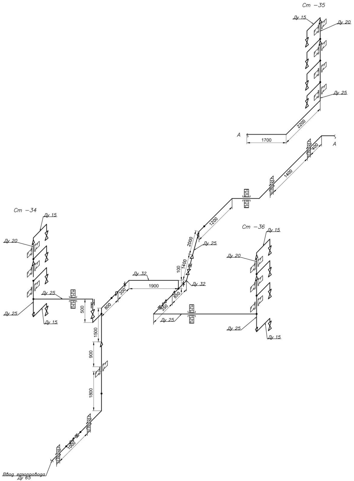
АксонOMETрическая схема внутридомового газового оборудования по адресу: Владимирская обл., Кольчугинский р-н, г. Кольчугино, ул. 50 лет Октября, д. 15 (подъезд 14)
