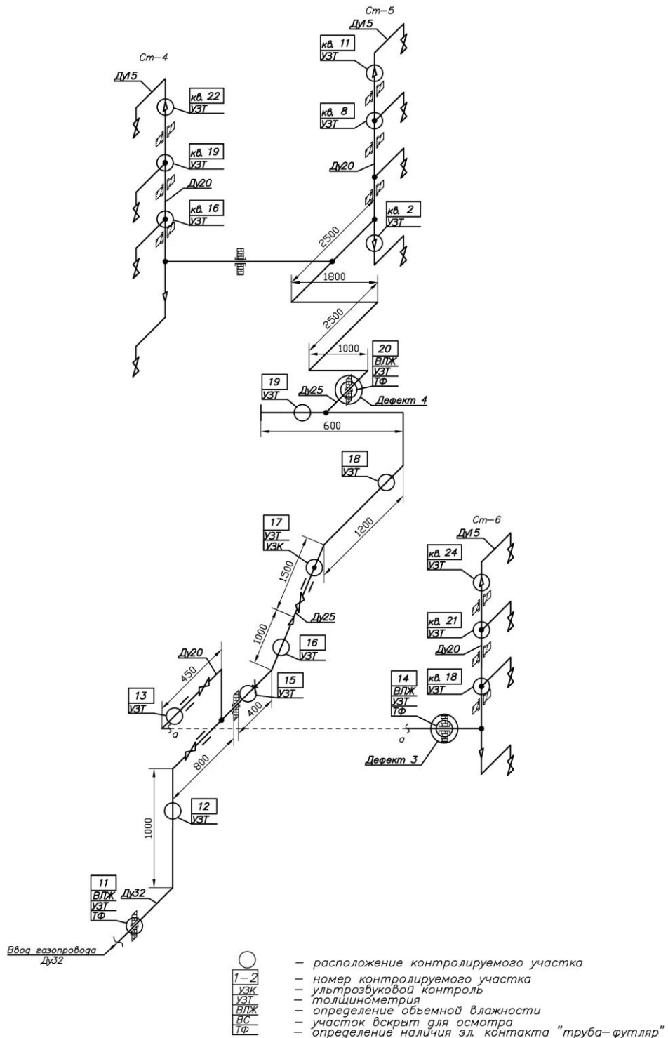
Схема неразрушающего контроля внутридомового газового оборудования по адресу: Владимирская обл., г. Кольчугинский р-н, Кольчугино, ул. Фурманова, д. 17 а (подъезд 2)
