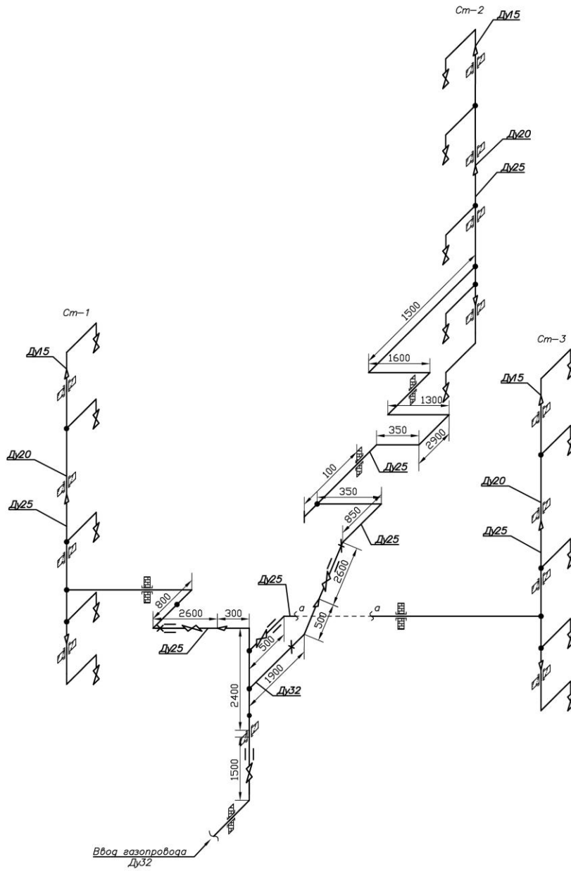
АксонOMETрическая схема внутридомового газового оборудования по адресу : Владимирская обл., Кольчугинский р-н, г. Кольчугино, ул. Коллективная, д. 47 (подъезд 1)
