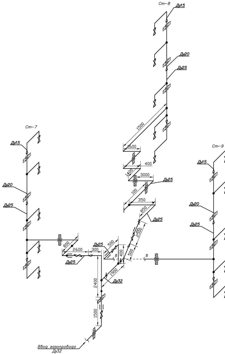
АксонOMETрическая схема внутридомового газового оборудования по адресу: Владимирская обл., Кольчугинский р-н, г. Кольчугино, ул. Коллективная, д. 47 (подъезд 3)
