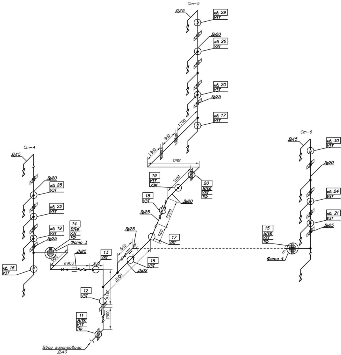
Схема неразрушающего контроля внутридомового газового оборудования по адресу: Владимирская обл., Кольчугинский р-н, г. Кольчугино, ул. Веденева, д. 2 (подъезд 2)
