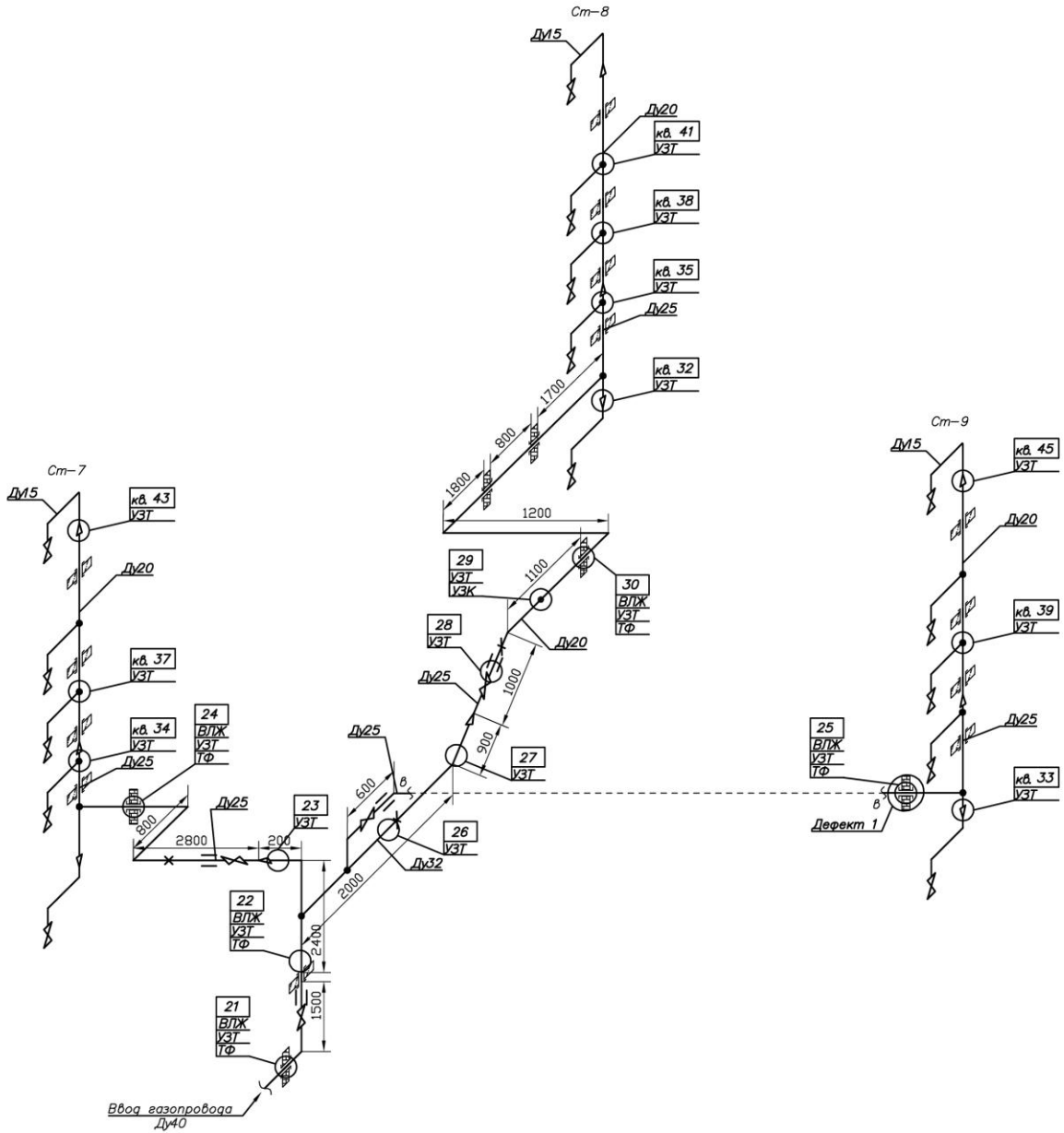
Схема неразрушающего контроля внутридомового газового оборудования по адресу: Владимирская обл., Кольчугинский р-н, г. Кольчугино, ул. Веденева, д. 2 (подъезд 3)
