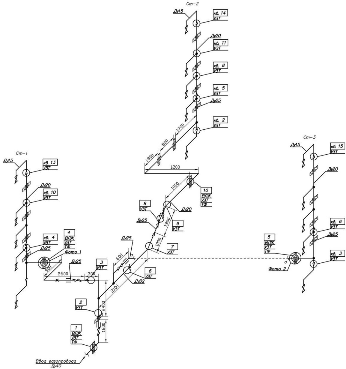
Схема неразрушающего контроля внутридомового газового оборудования по адресу: Владимирская обл., Кольчугинский р-н, г. Кольчугино, ул. Веденева, д. 2 (подъезд 1)
