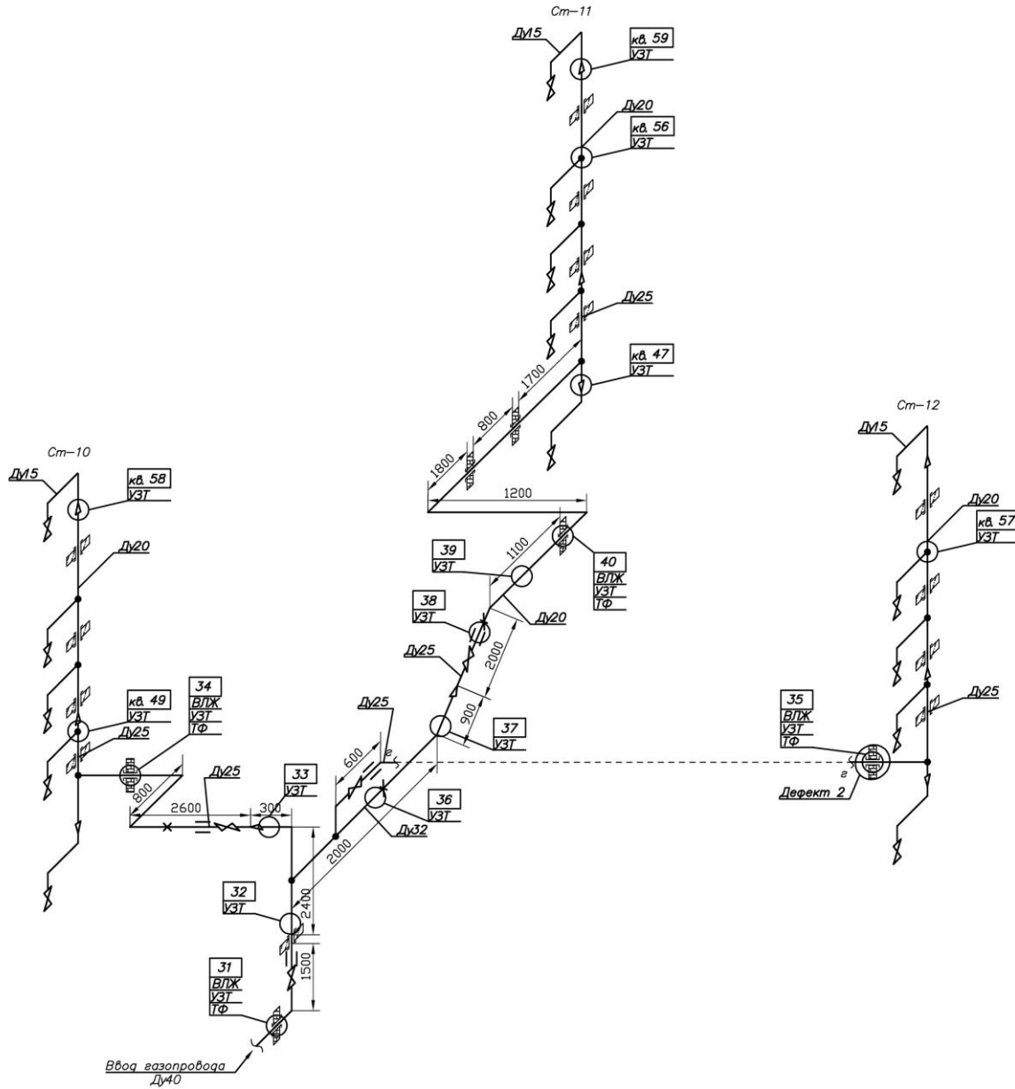
Схема неразрушающего контроля внутридомового газового оборудования по адресу: Владимирская обл., Кольчугинский р-н, г. Кольчугино, ул. Веденеева, д. 2 (подъезд 4)
