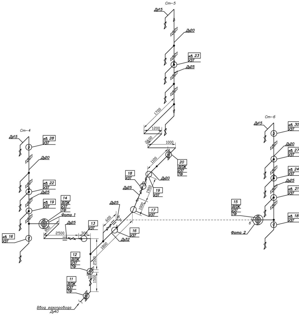
Схема неразрушающего контроля внутридомового газового оборудования по адресу: Владимирская обл., Кольчугинский р-н, г. Кольчугино, ул. Веденева, д. 6 (подъезд 2)
