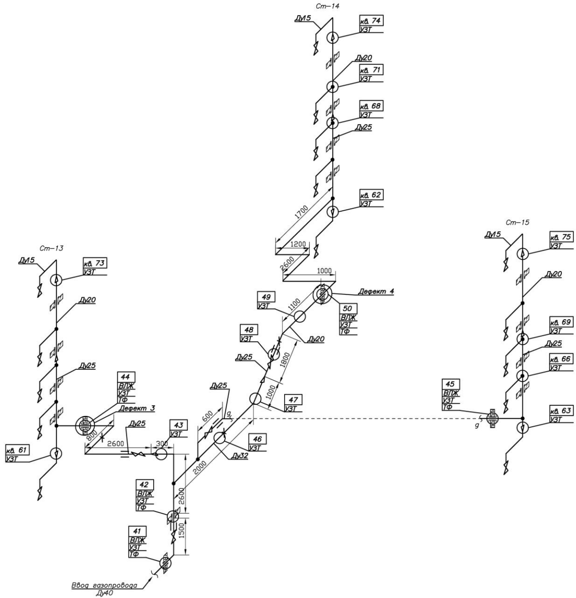
Схема неразрушающего контроля внутридомового газового оборудования по адресу: Владимирская обл., Кольчугинский р-н, г. Кольчугино, ул. Веденева, д. 6 (подъезд 5)
