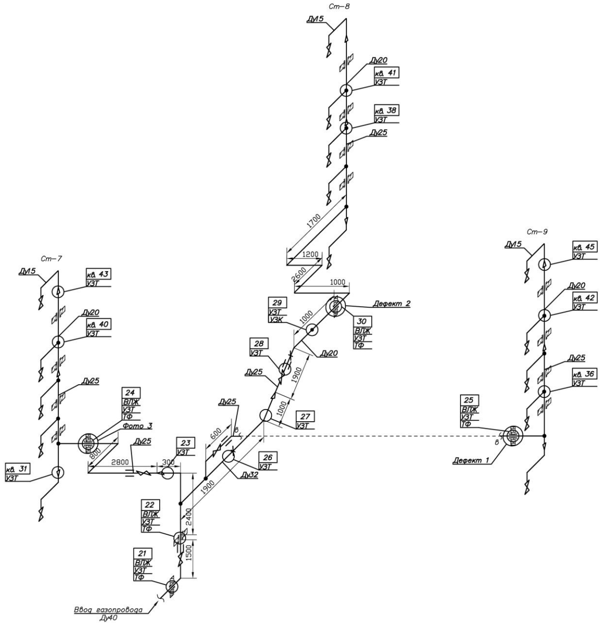
Схема неразрушающего контроля внутридомового газового оборудования по адресу: Владимирская обл., Кольчугинский р-н, г. Кольчугино, ул. Веденева, д. 6 (подъезд 3)
