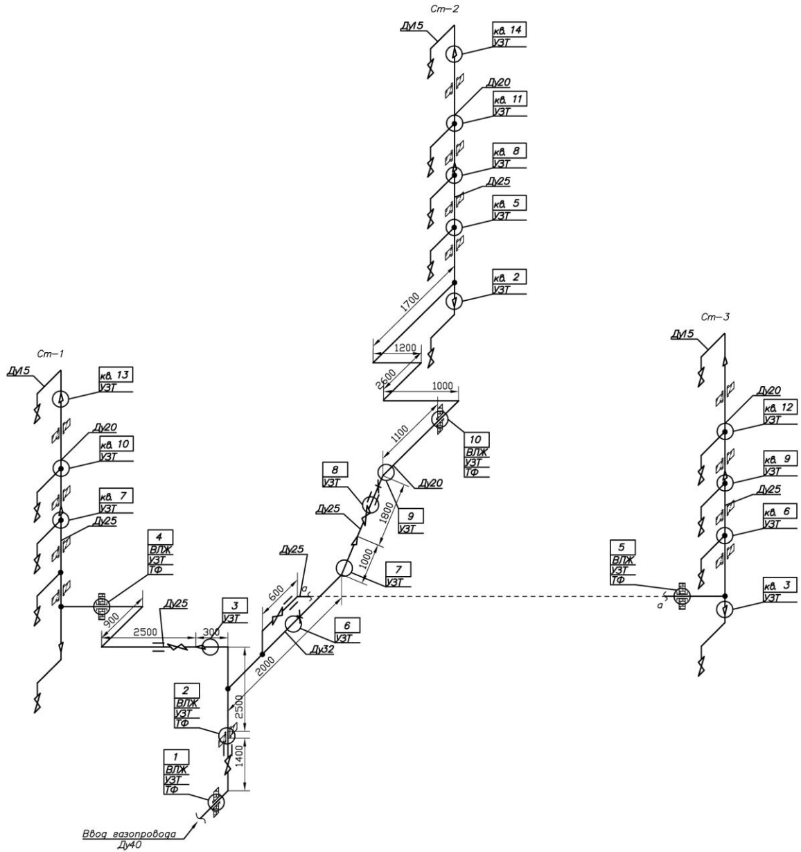
Схема неразрушающего контроля внутридомового газового оборудования по адресу: Владимирская обл., Кольчугинский р-н, г. Кольчугино, ул. Веденева, д. 6 (подъезд 1)
