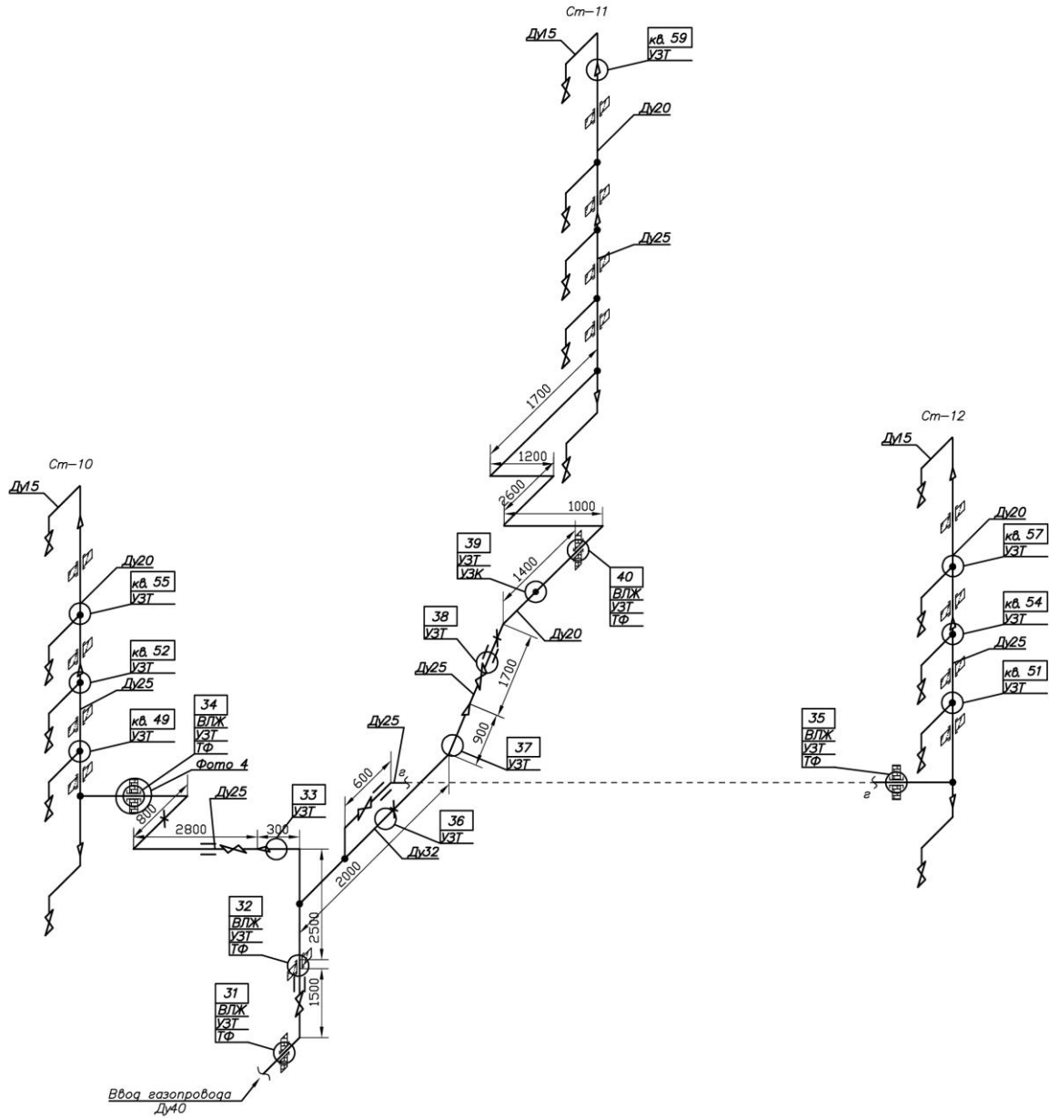
Схема неразрушающего контроля внутридомового газового оборудования по адресу: Владимирская обл., Кольчугинский р-н, г. Кольчугино, ул. Веденева, д. 6 (подъезд 4)
