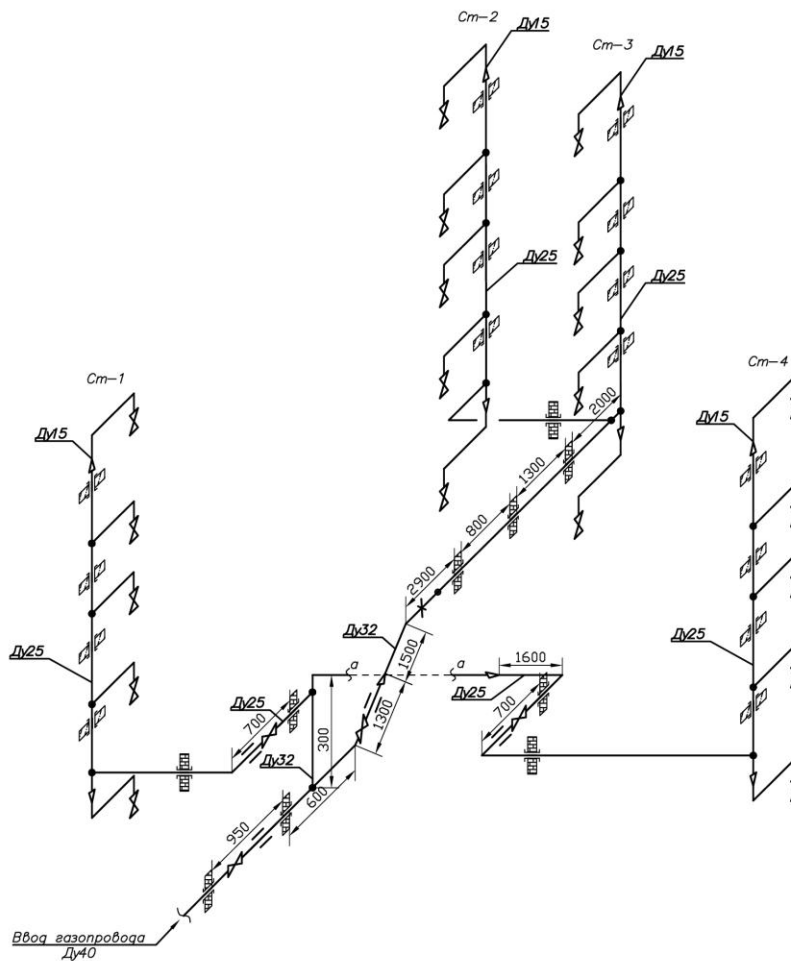
АксонOMETрическая схема внутридомового газового оборудования по адресу: Владимирская обл., Кольчугинский р-н, г. Кольчугино, ул. 50 лет Октября, д. 24 (подъезд 1)
