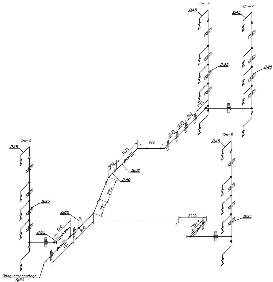
АксонOMETрическая схема внутридомового газового оборудования по адресу: Владимирская обл., Кольчугинский р-н, г. Кольчугино, ул. Алексеева, д. 1 а (подъезд 2)
