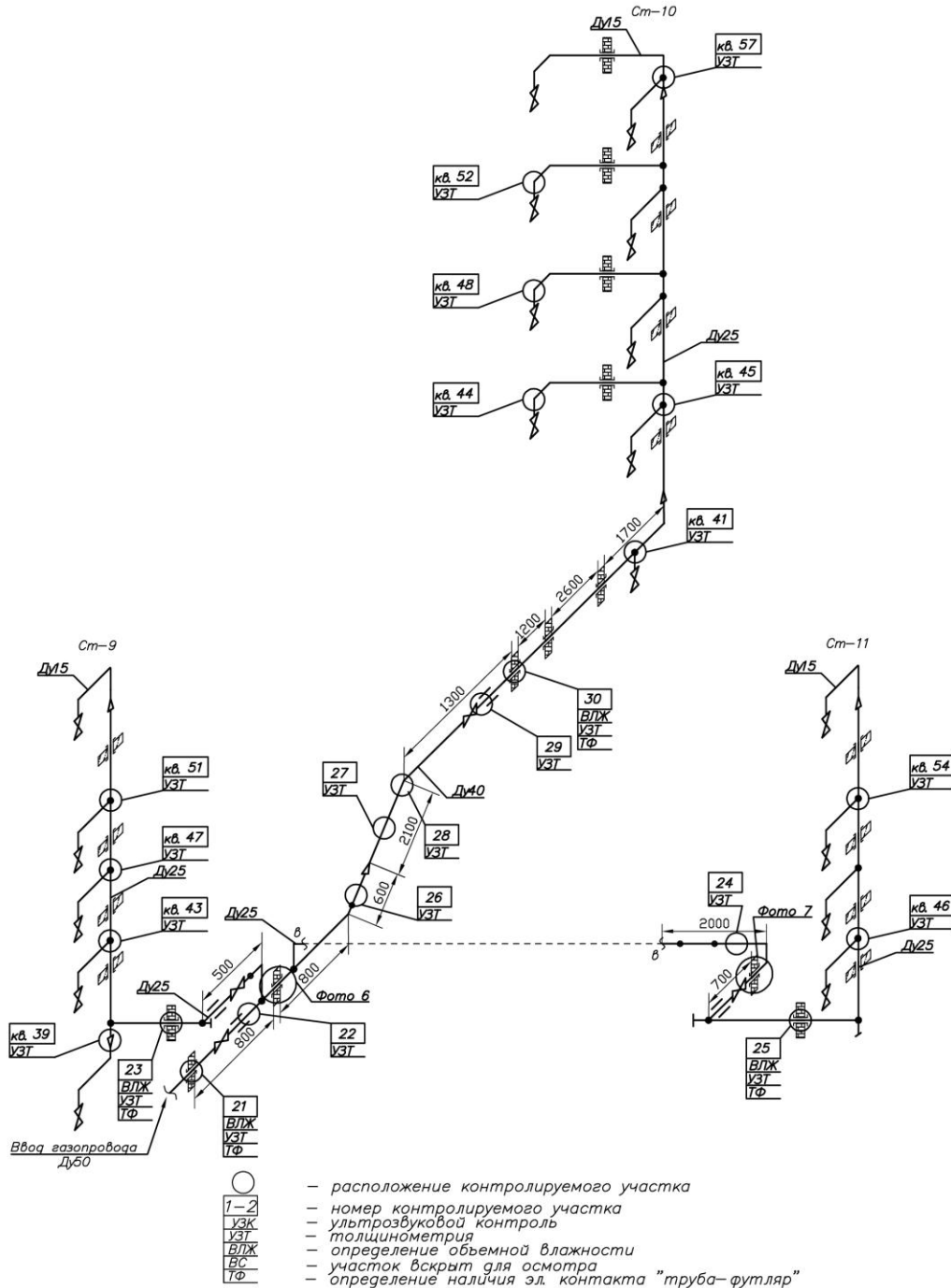
Схема неразрушающего контроля внутридомового газового оборудования по адресу: Владимирская обл., Кольчугинский р-н, г. Кольчугино, ул. Алексеева, д. 1 а (подъезд 3)
