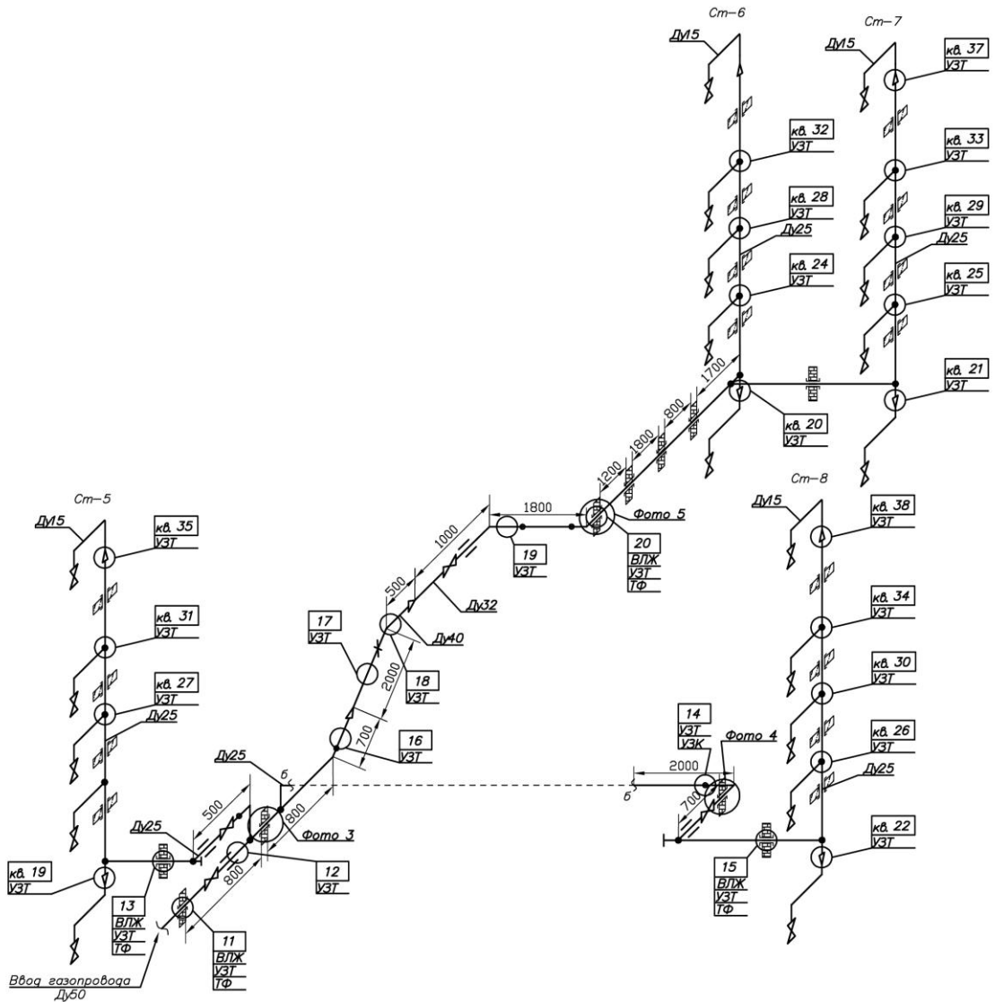
Схема неразрушающего контроля внутридомового газового оборудования по адресу: Владимирская обл., Кольчугинский р-н, г. Кольчугино, ул. Алексеева, д. 1 а (подъезд 2)
