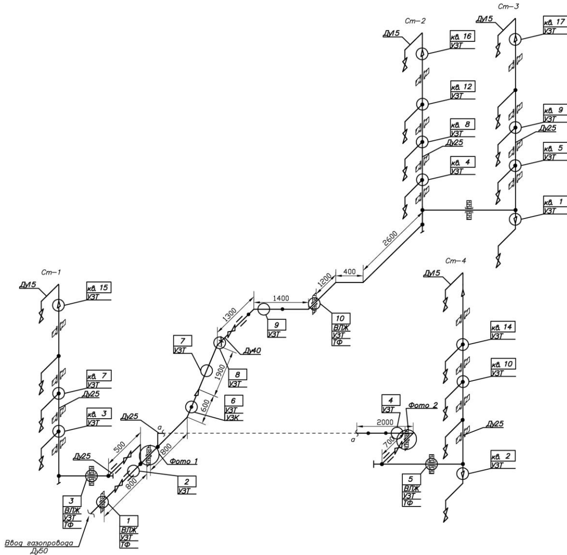
Схема неразрушающего контроля внутридомового газового оборудования по адресу: Владимирская обл., Кольчугинский р-н, г. Кольчугино, ул. Алексеева, д. 1 а (подъезд 1)
