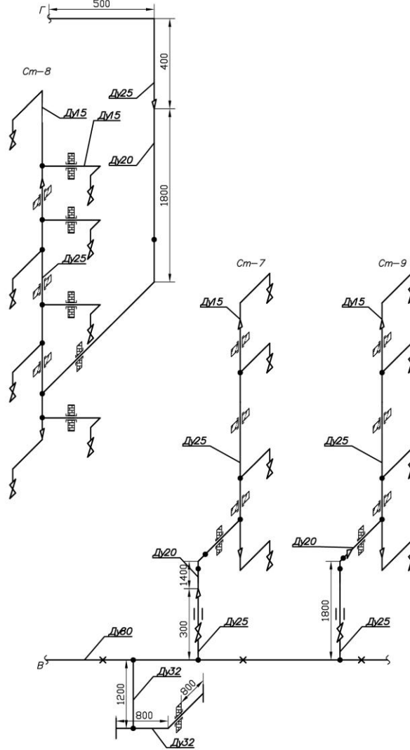
АксонOMETрическая схема внутридомового газового оборудования по адресу: Владимирская обл., Кольчугинский р-н, г. Кольчугино, ул. Дружбы, д. 15 (подъезд 3)
