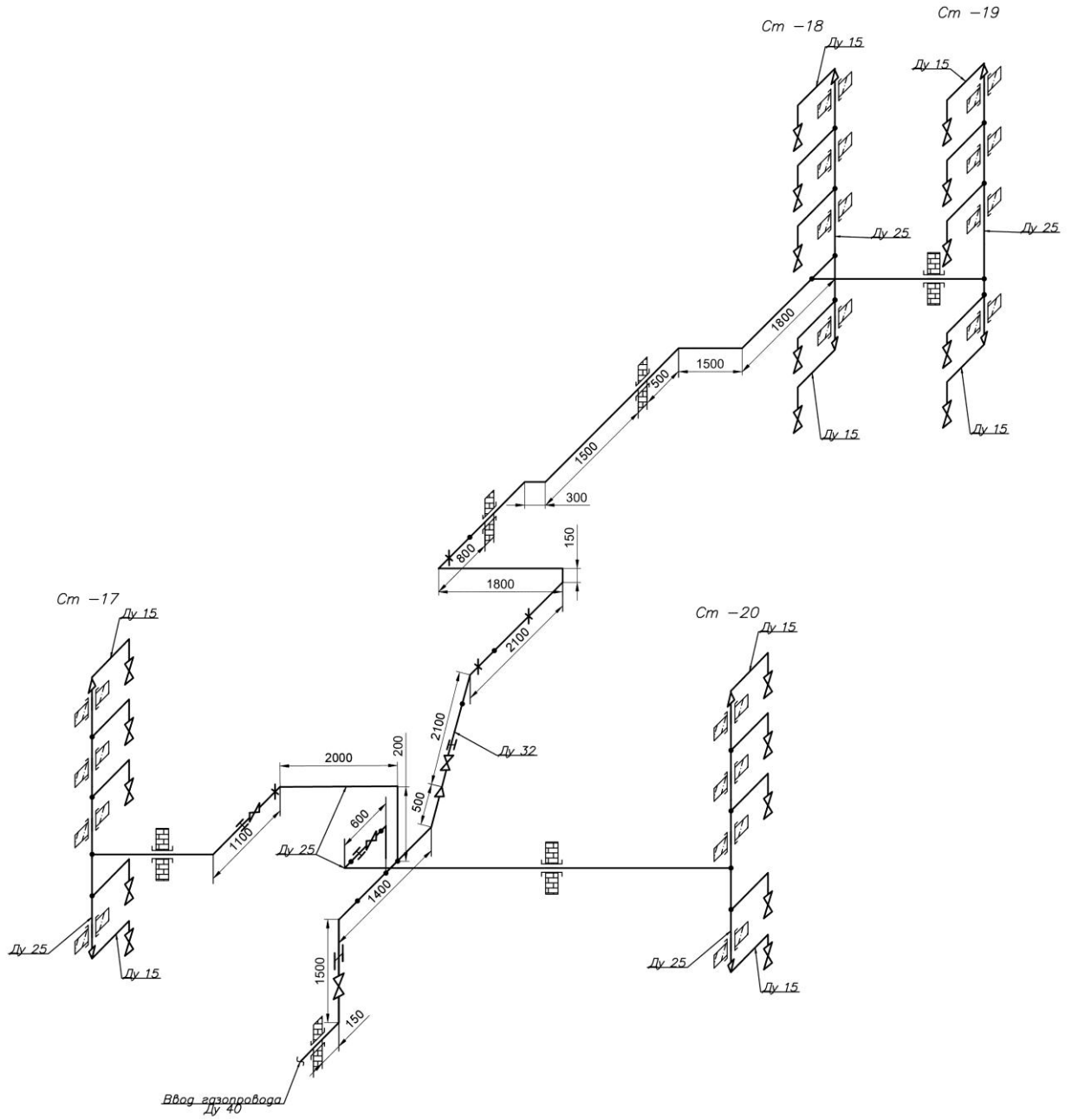
АксонOMETрическая схема внутридомового газового оборудования по адресу: Владимирская обл., Кольчугинский р-н, г. Кольчугино, ул. Дружбы, д. 31 (подъезд 6)
