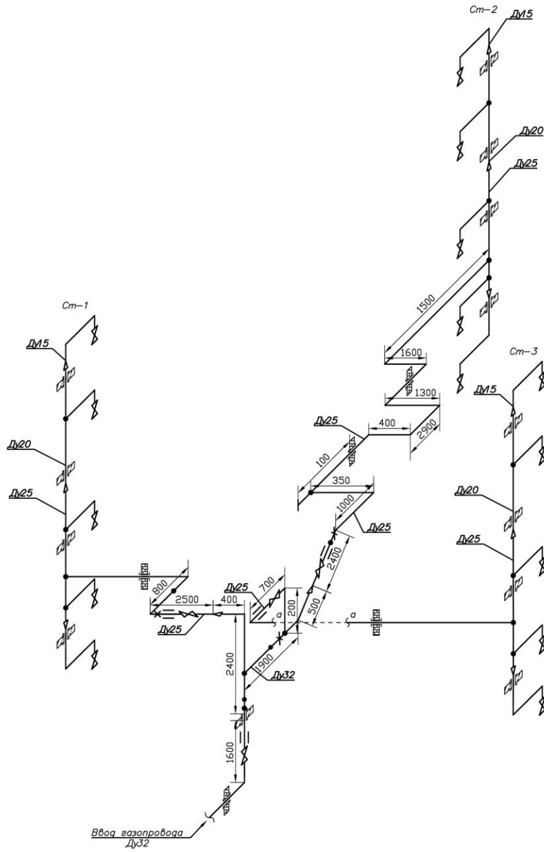
АксонOMETрическая схема внутридомового газового оборудования по адресу : Владимирская обл., Кольчугинский р-н, г. Кольчугино, ул. Коллективная, д. 39 (подъезд 1)
