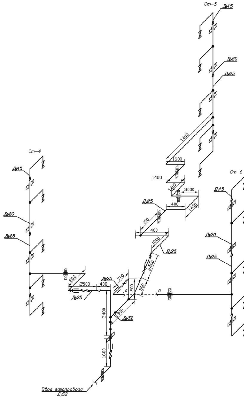
АксонOMETрическая схема внутридомового газового оборудования по адресу: Владимирская обл., Кольчугинский р-н, г. Кольчугино, ул. Коллективная, д. 39 (подъезд 2)
