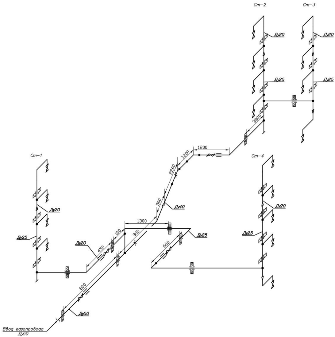
АксонOMETрическая схема внутридомового газового оборудования по адресу : Владимирская обл., Кольчугинский р-н, г. Кольчугино, ул. Мира, д. 3 (подъезд 1)
