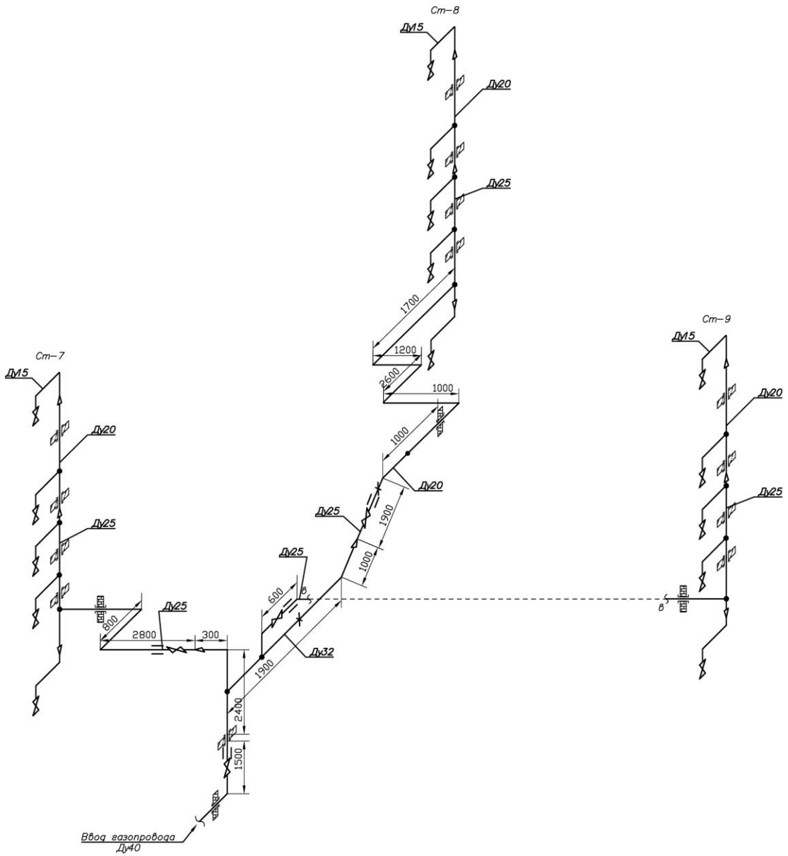
АксонOMETрическая схема внутридомового газового оборудования по адресу : Владимирская обл., Кольчугинский р-н, г. Кольчугино, ул. Веденева, д. 6 (подъезд 3)
