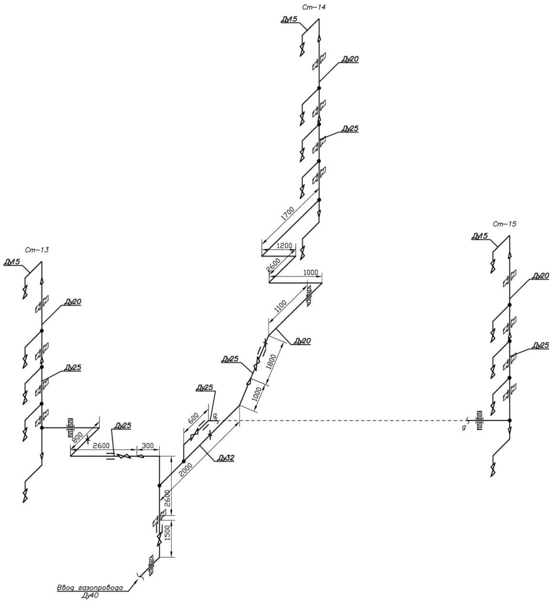
АксонOMETрическая схема внутридомового газового оборудования по адресу: Владимирская обл., Кольчугинский р-н, г. Кольчугино, ул. Веденева, д. 6 (подъезд 5)
